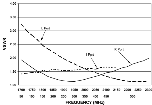
VSWR
