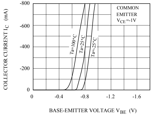
I_C - V_{BE}
